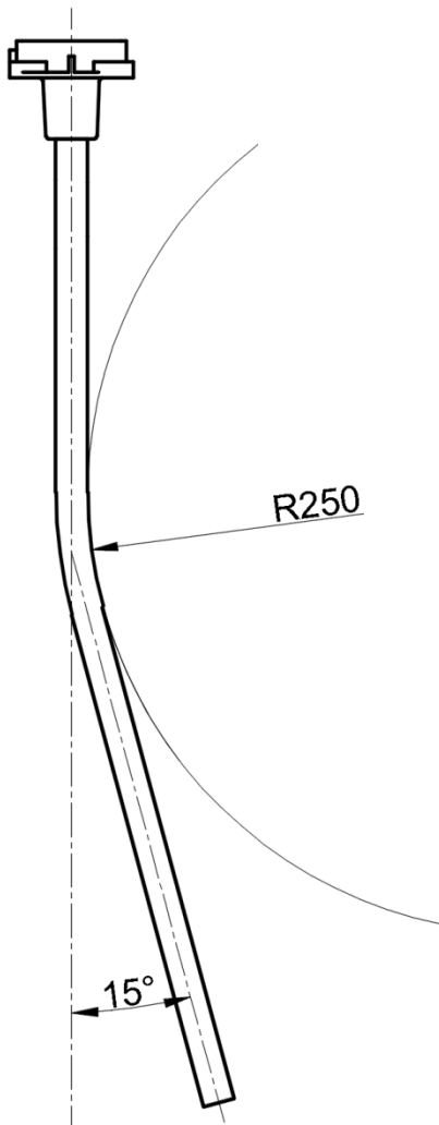
Рисунок 5. Изгиб трубки датчика.
