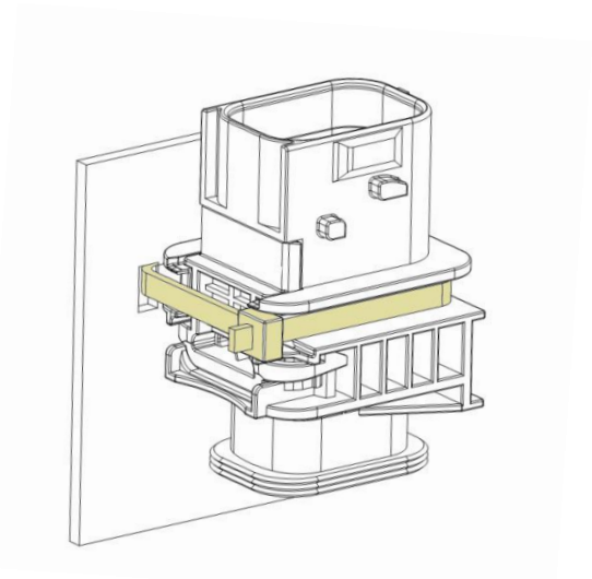
Рисунок 7. Крепление разъема.
