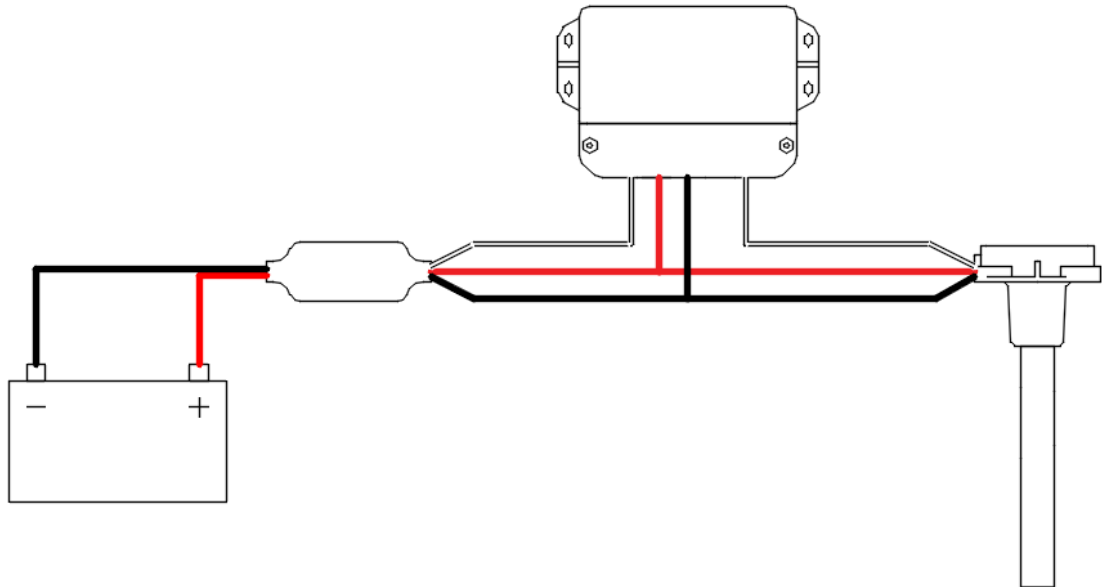
Рисунок 9. Схема подключения с использованием частотного сигнала и общего источника питания.
